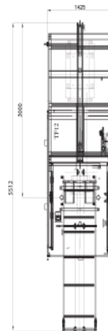
Прямой выход лотка
